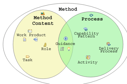
5.12. Irudia. UMA metodologiako metodoaren eta prozesuaren kontzeptuak.
