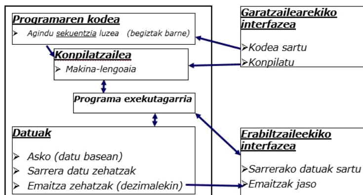
3.5. Irudia. Programazio tradizionalaren eskema.
